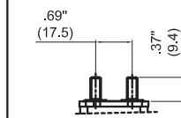
L Two 10-32 studs: (AUX&BAT)
